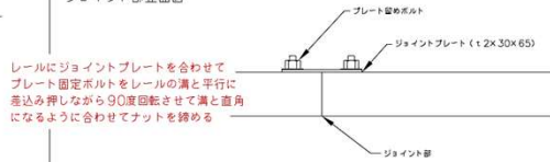
ジョイント部立面図
