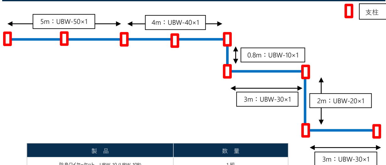
パターン①：アルティマ防鳥ワイヤーセット (ワイヤー線径φ1.2)
