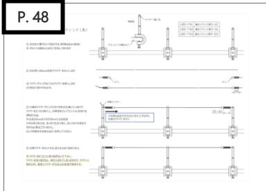
E-2 支柱 UBS-FN Φ0.8 UBWM□-ル + UBWM(B)グリップ
