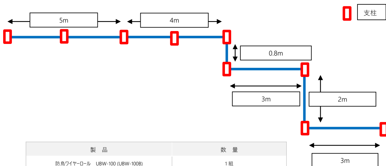
パターン②：防鳥ワイヤーロール+グリップ内蔵バネフック (ワイヤー線径φ1.2)
