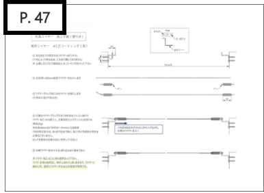
C-2 支柱 UBS-T00 Φ1.2 UBW□-ル + UBW(B)グリップ
