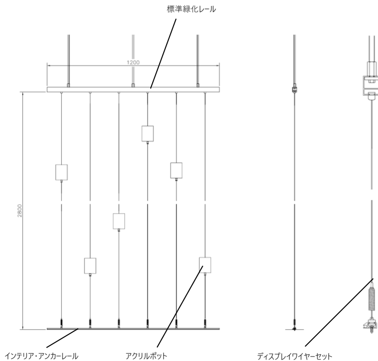
アルティマグリュネ・フェenster【ディスプレイ】製品組み合わせ一覧表_2-1：ビス止め取付タイプ：アルミ製緑化レール仕様
